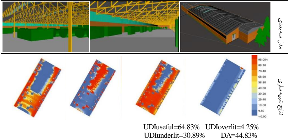
شکل ۴. نمودار از بالا به پایین مدل سه بعدی کارگاه از دید پرند، فضای داخلی کارگاه DA، (UDIunderlit)، (UDIuseful)، (UDIoverlit)، در شرایط وضع موجود (نویسندگان).
