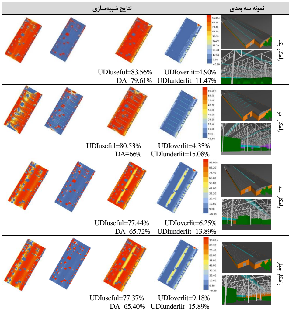
شکل ۴. نمودار از راست به چپ، مدل سه بعدی کارگاه از دید پرنده، فضای داخلی کارگاه، DA، (UDUnderlit)، (UDUseful)، (UDloverlit)، شرایط راهکارها (نویسندگان).
