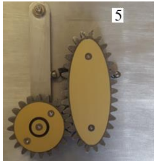
شکل ۱۳. سیکل کامل چرخشی مکانیزم چرخنده‌ای به ترتیب از تصاویر ۱ تا ۵ (در جهت ساعتگرد دوران چرخنده محرک بیضوی).
