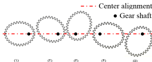
شکل ۳. نحوه حرکت یک چرخدنده بیضوی تک‌گوشه در یک سیکل کامل دورانی (جهت ساعتگرد).
