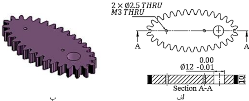
شکل ۷. چرخنده بیضوی تک گوشه: الف- نمای بالا و برش خورده، ب- تصویر مجسم ایزومتریک (ابعاد به میلیمتر).
