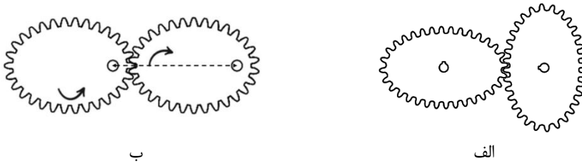
شکل ۱. نحوه درگیری دو چرخدنده: الف- بیضوی دوگوشه و ب- بیضوی تک‌گوشه.
