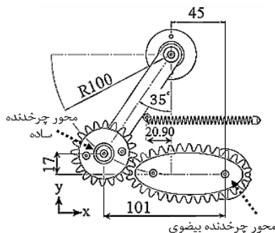
شکل ۱۰. درگیری چرخنده ساده و بیضوی در حداکثر فاصله ممکن بین شفت‌ها و میزان افزایش طولی فنر (ابعاد به میلیمتر).
