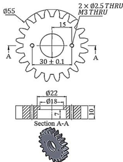
شکل ۶. چرخدنده ساده طراحی شده (ابعاد به میلیمتر - محدوده تolerانس با درجه کیفی IT۷ در تمام ابعاد نقشه تابع: ISO ۲۸۶-۱).
