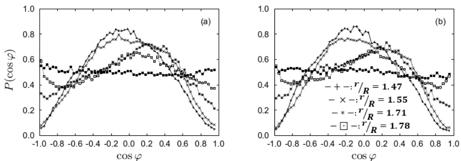
شکل ۱۰. جهت‌گیری ممان دوقطبی در فواصل مختلف از دیواره‌های نانولوله گرافدین (۴ و ۴) بدون ممان چهارقطبی (b) با ممان چهارقطبی.
