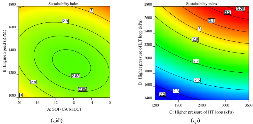
شکل ۹. الف) اثرات N و SOI بر شاخص پایداری، در حالی که HPHT=2400 kPa و HPLT=2100 kPa ب) اثرات HPLT و HPHT بر شاخص پایداری، در حالی که SOI=-10 CA bTDC و N=1400 RPM
