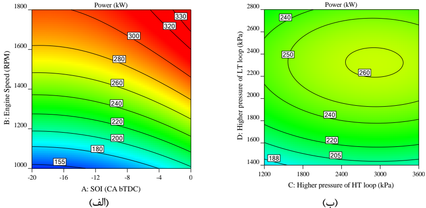
شکل ۶. اثرات SOI و N بر توان تولیدی، در حالی که HPHT=2400 kPa و HPLT=2100 kPa (ب) اثرات HPHT و HPLT بر توان تولیدی، در حالی که SOI=-10 CA bTDC و N=1400 RPM
