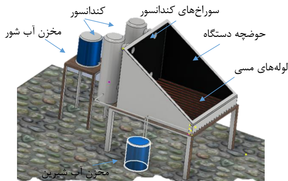
شکل ۱. طرح‌واره آب شیرین‌کن پیشنهادی.
