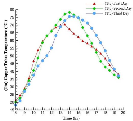
شکل ۱۰. دمای داخل کندانسورها در روزها آزمایش.
