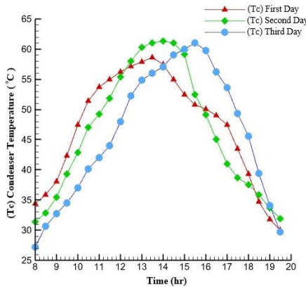
شکل ۹. دمای لوله‌های مسی در روزهای آزمایش.
