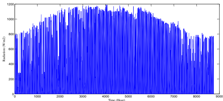
شکل ۲. منحنی تابش سالیانه در شهر کرمان.
