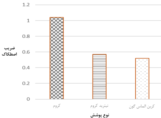
شکل ۶. میانگين ضریب اصطکاک اندازه‌گیری شده برای سه پوشش کروم سخت، نیتريد کروم و کربن الماس گون بعد از ۵۰۰ متر
