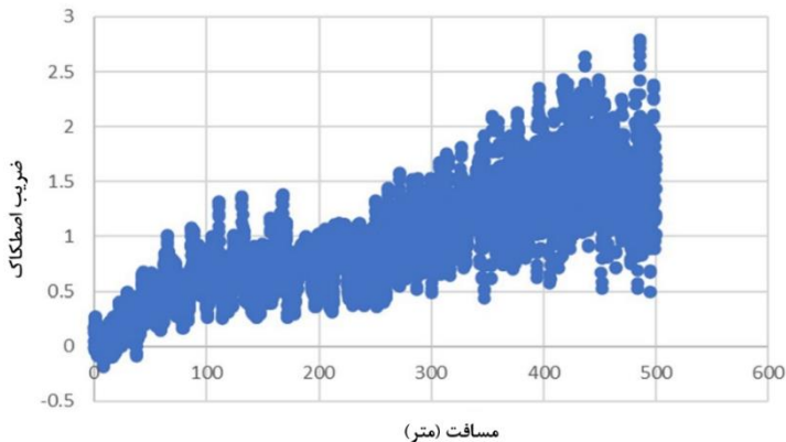
شکل ۴. ضریب اصطکاک بر حسب فاصله طی شده توسط نمونه رینگ با پوشش کروم سخت
