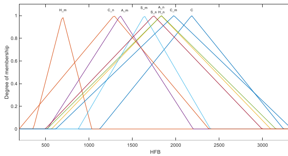
شکل ۲. توابع عضویت متغیر ورودی HFB
