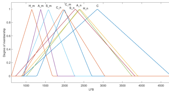
شکل ۳. توابع عضویت متغیر ورودی LFB
