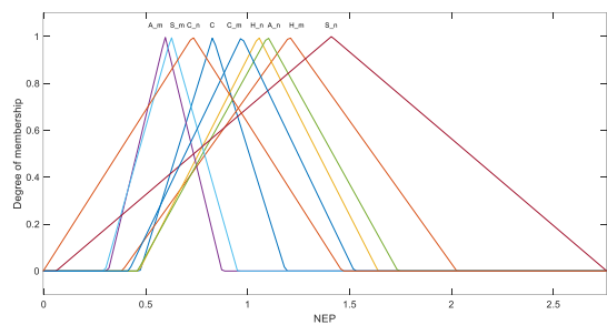
شکل ۵. توابع عضویت متغیر ورودی NEP .
