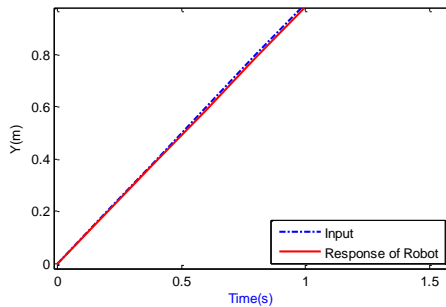
شکل ۱۰. پاسخ کنترل‌گر PID به تابع شیب.
