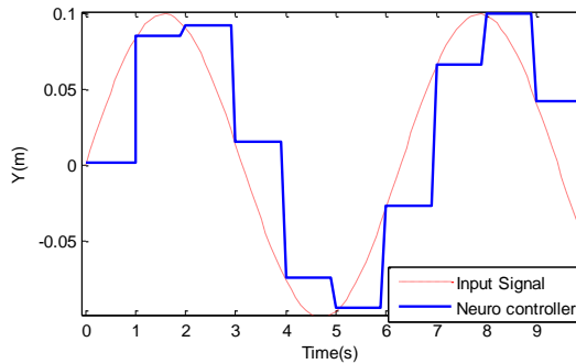
شکل ۱۳. خروجی کنترلر گر تطبیقی شبکه عصبی نسبت به تابع سینوسی.
