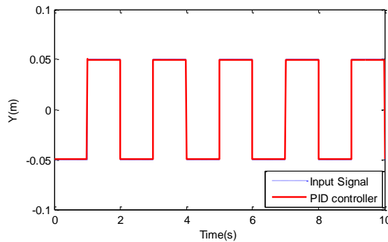
شکل ۱۶. پاسخ ربات مجهز به کنترل‌کننده PID به موج مربعی.
