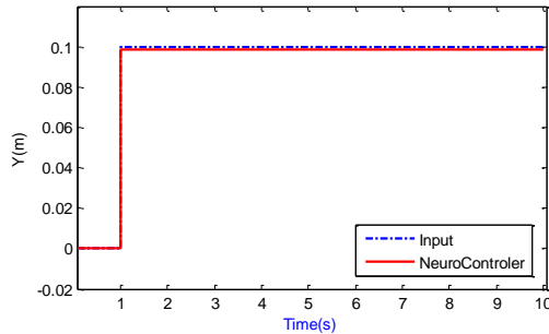
شکل ۹. پاسخ کنترل‌کننده وقفی شبکه عصبی.
