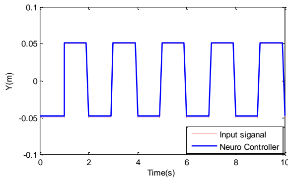
شکل ۱۷. پاسخ تولید شده ربات مجهز به کنترل‌گر وفقی شبکه عصبی به موج مربعی.
