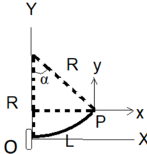
شکل ۳. موقعیت مکانی انتهایی بازو و شعاع انحنا.
