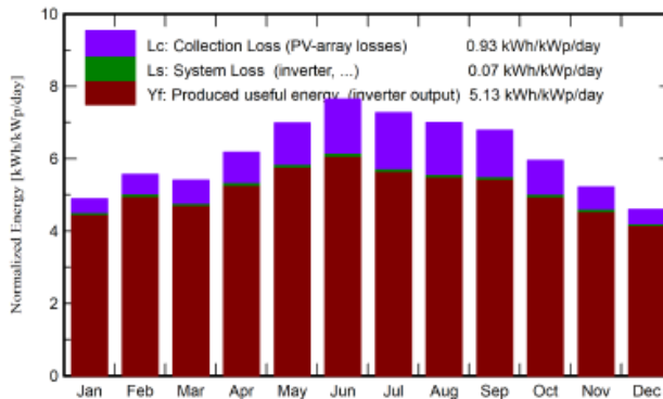
شکل ۱۸. میزان تولید نرمال شده سیستم STAP
