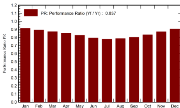
شکل ۱۹. ضریب عملکرد سیستم STAP.
