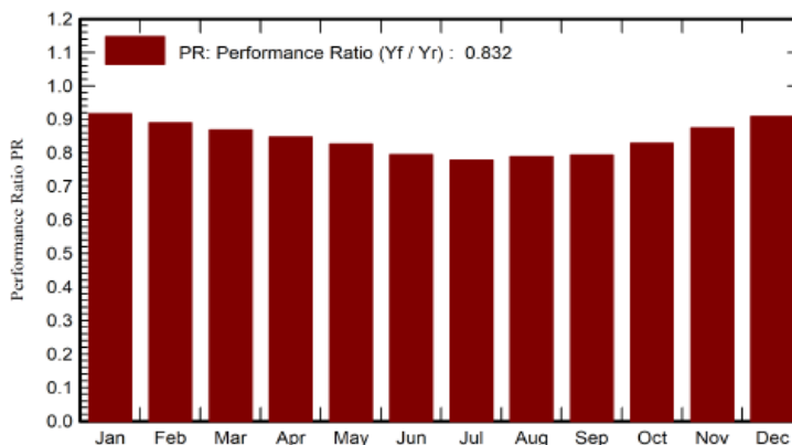
شکل ۱۵. ضریب عملکرد سیستم TTP.
