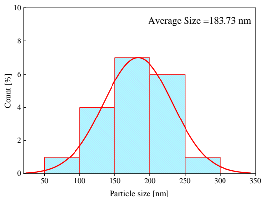
شکل ۳. نمودار توزیع اندازه ذرات میکروسکوپی \text{TiO}_2 .
