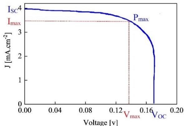
شکل ۶. نمودار جریان-ولتاژ سلول خورشیدی حساس‌شده با رنگ‌دانه حنای ساده بر پایه الکترولیت نیمه-جامد و الکتروود مقابل اکسید زیرکونیوم/اکسید تنگستن.
