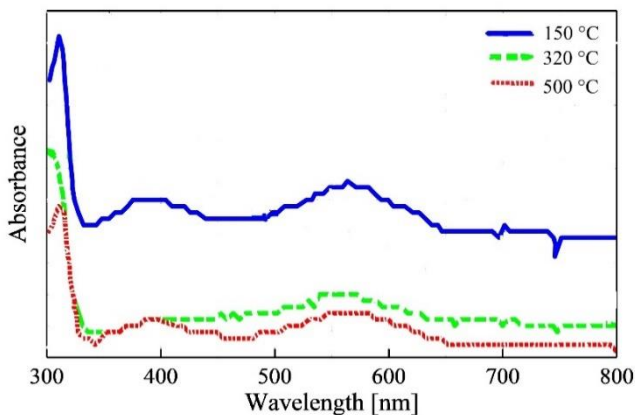
شکل ۵. طیف جذبی فوتوآند در دماهای بازپخت مختلف.
