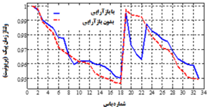
شکل ۱۰. تاثیر روش پیشنهادی بر منحنی ولتاژ (مورد ۴).
