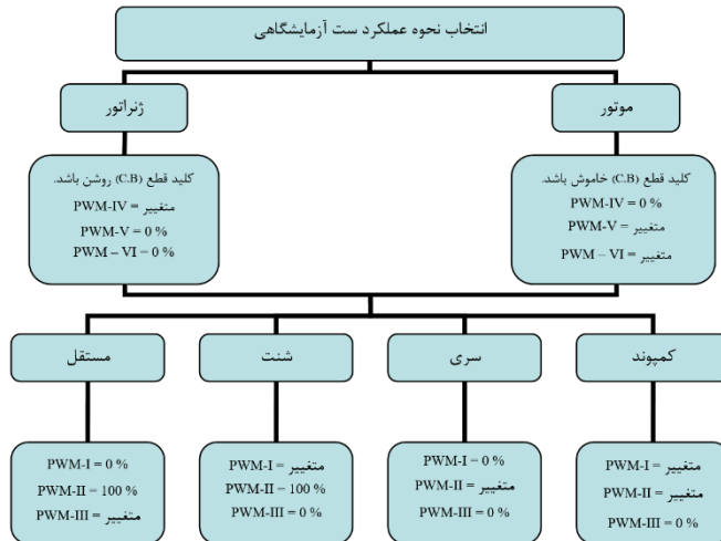
شکل ۱۱. فلوجارت عملکرد آزمایشگاه
