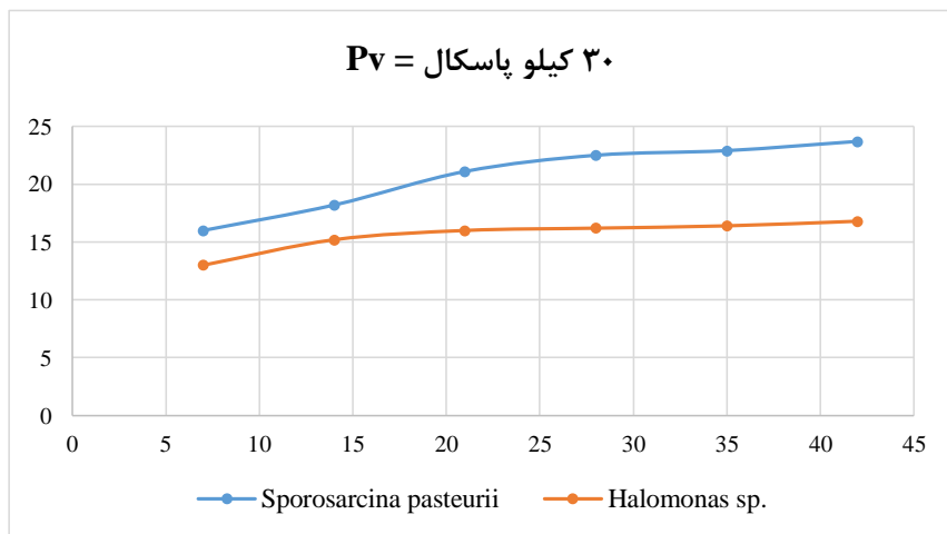
شکل ۴. مقاومت برشی خاک تحت تنش ۳۰ کیلو پاسکال در طی ۴۲ روز، محور x نشانگر تنش برشی، محور Y زمان بر حسب روز.
