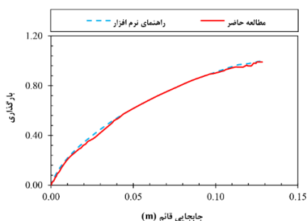
شکل ۳. نمودار بار-جابجایی.
