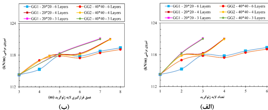
الف) براساس تعداد لایه‌های ژئوگرید، ب) براساس عمق قرارگیری و فواصل قائم لایه‌های ژئوگرید
