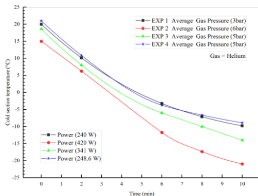
شکل ۱۶. دیاگرام دما- زمان برای آزمایش‌های انجام‌شده با گاز هلیوم در فشارهای مختلف و حالت موتور خنک‌کننده [۲۳]
