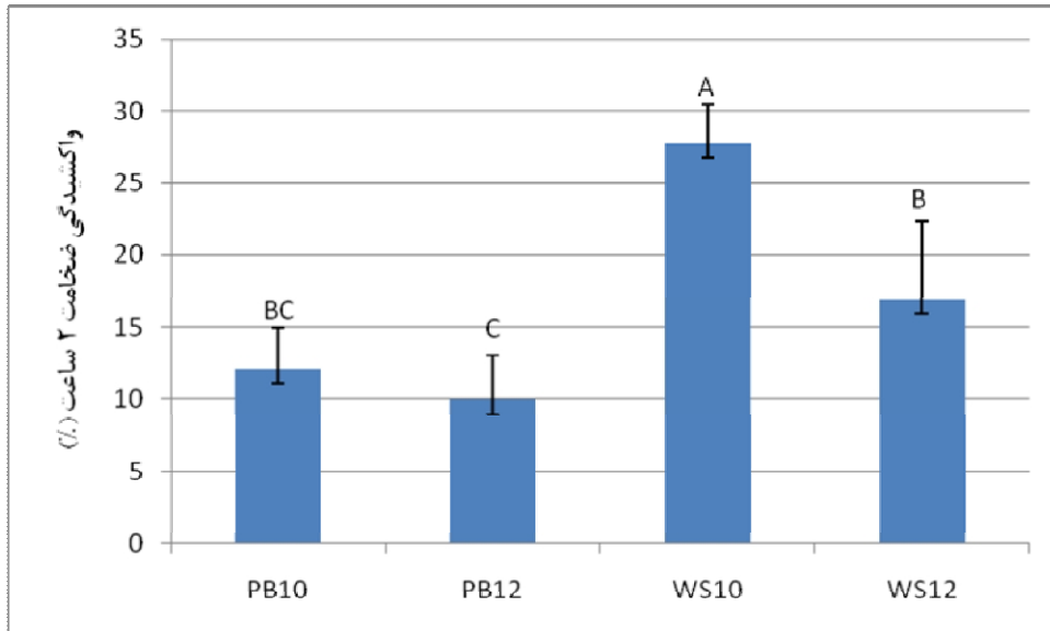
شکل 3. اثر نوع ماده لیگنوسولوزی و درصد چسب بر واکنش پذیری ضخامت 2 ساعت
