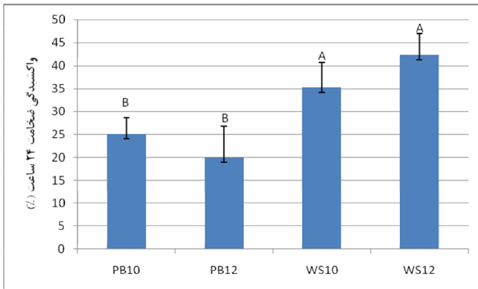
شکل 4. اثر نوع ماده لیگنوسولوزی و درصد چسب بر واکنش پذیری ضخامت 24 ساعت
