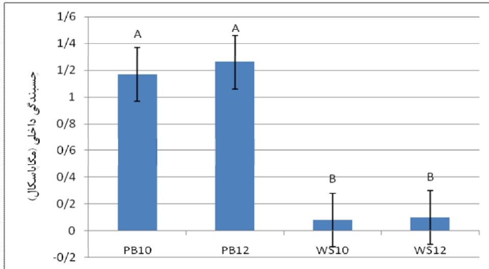
شکل 5. اثر نوع ماده لیگنوسولوزی و درصد چسب بر جسبندگی داخلی
