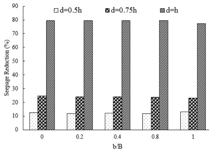
شکل 8. تأثیر جایگاه دیوار آب‌بند بر کاهش نشت
