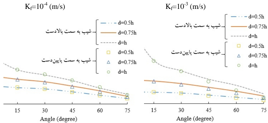
شکل 9. تأثیر زاویه دیوار آببند بر کاهش نشت
