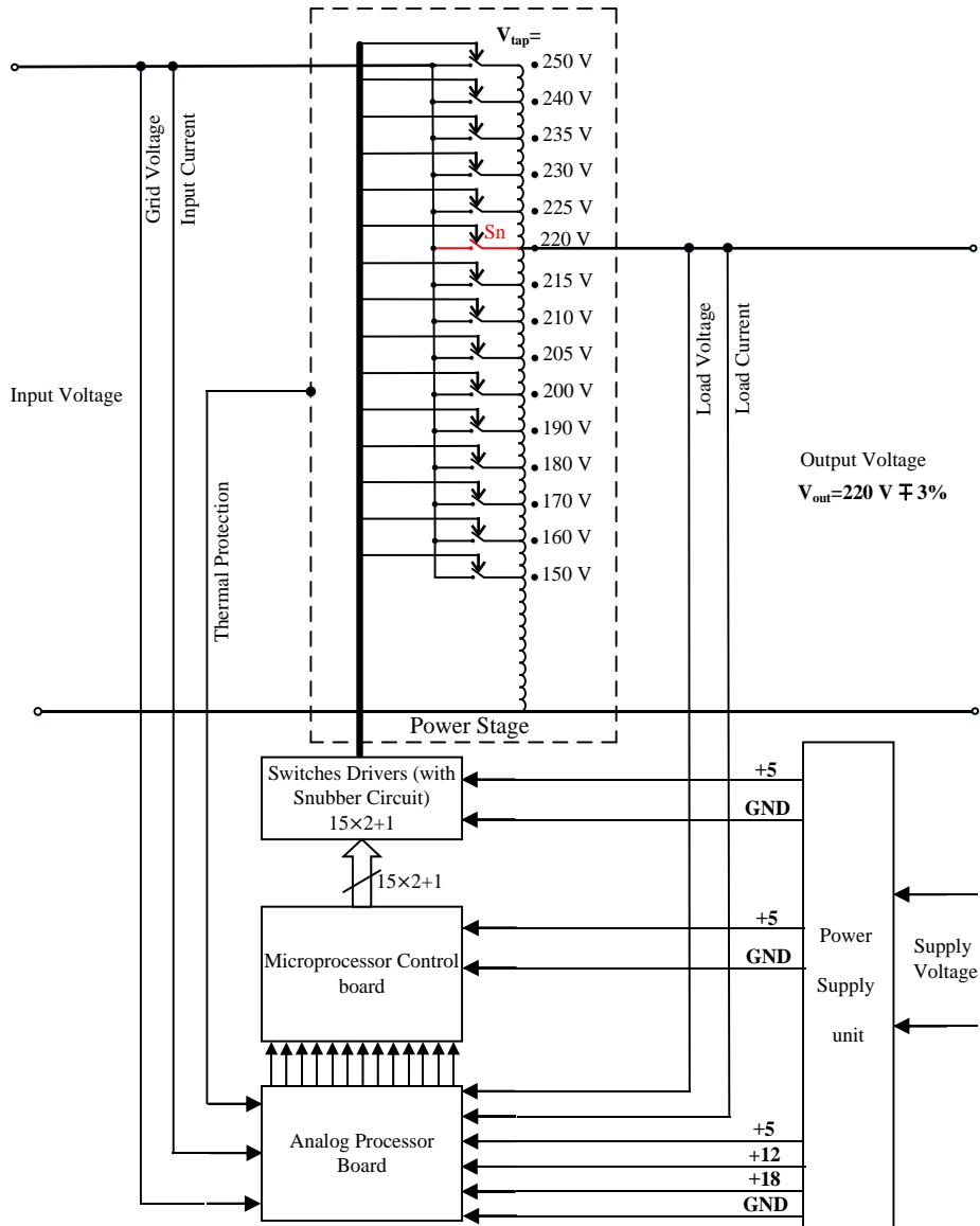
شکل ۳. شماتیک کلی کنترلی تنظیم کننده ولتاژ حالت جامد پیشنهادی.
