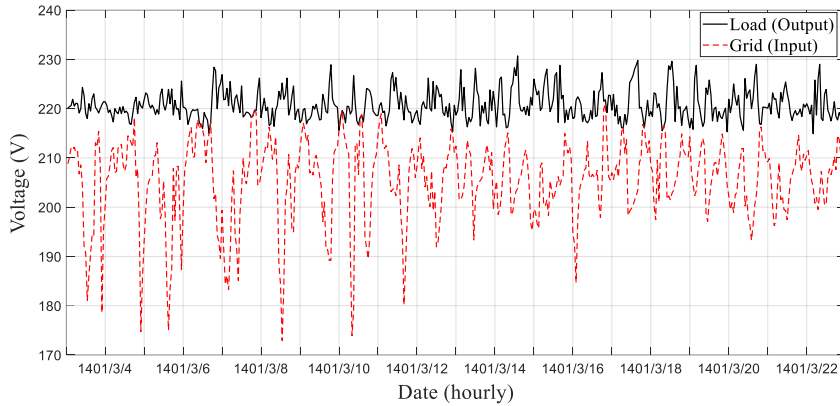
شکل ۱۱. ولتاژ ورودی و خروجی SSVR اندازه‌گیری شده در بازه خرداد ماه ۱۴۰۱.
